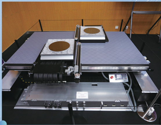
参展项目:光刻机气浮平面电机双工件台样机。
